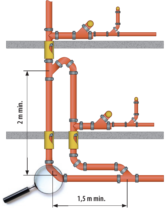
Resim 14 Dikey boru kavisi \geq 2m bypass borulu veya bypass borusu geçiş için toplama ve yeraltı borusuna giden bir dikey boru
