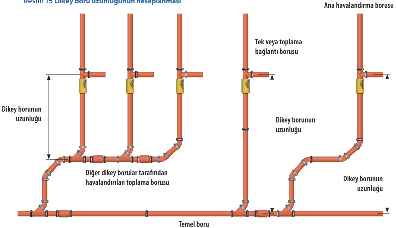
Resim 15 Dikey boru uzunluğunun hesaplanması
