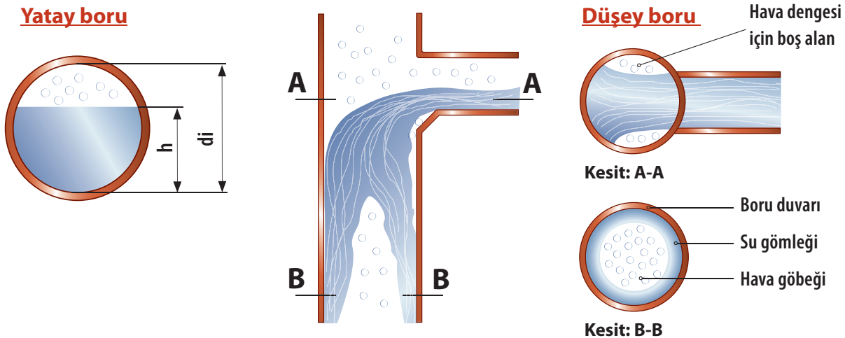
Resim 02 Çatal boru arkasındaki dikey borularda su gömleği ve hava göbeği oluşumu
