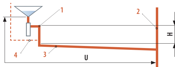
1 Bağlantı dirseği 2 Düşey boru 3 Bağlantı borusu 4 Havalandırma
