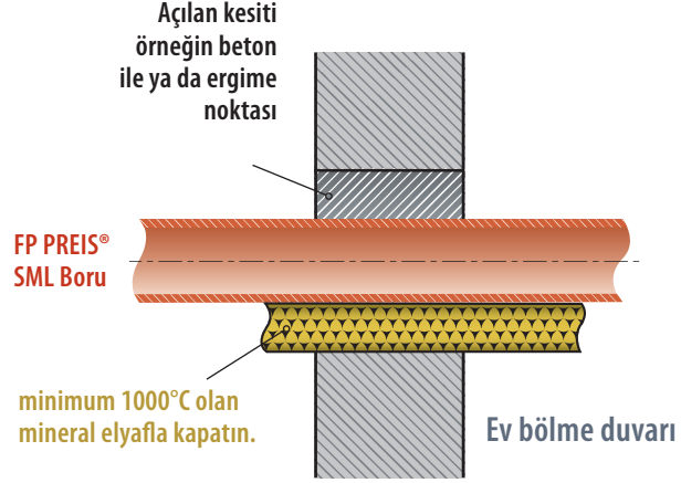
Resim 22 Yangından korunma açısından duvar boru hatları (yangın duvarları) talepleri
