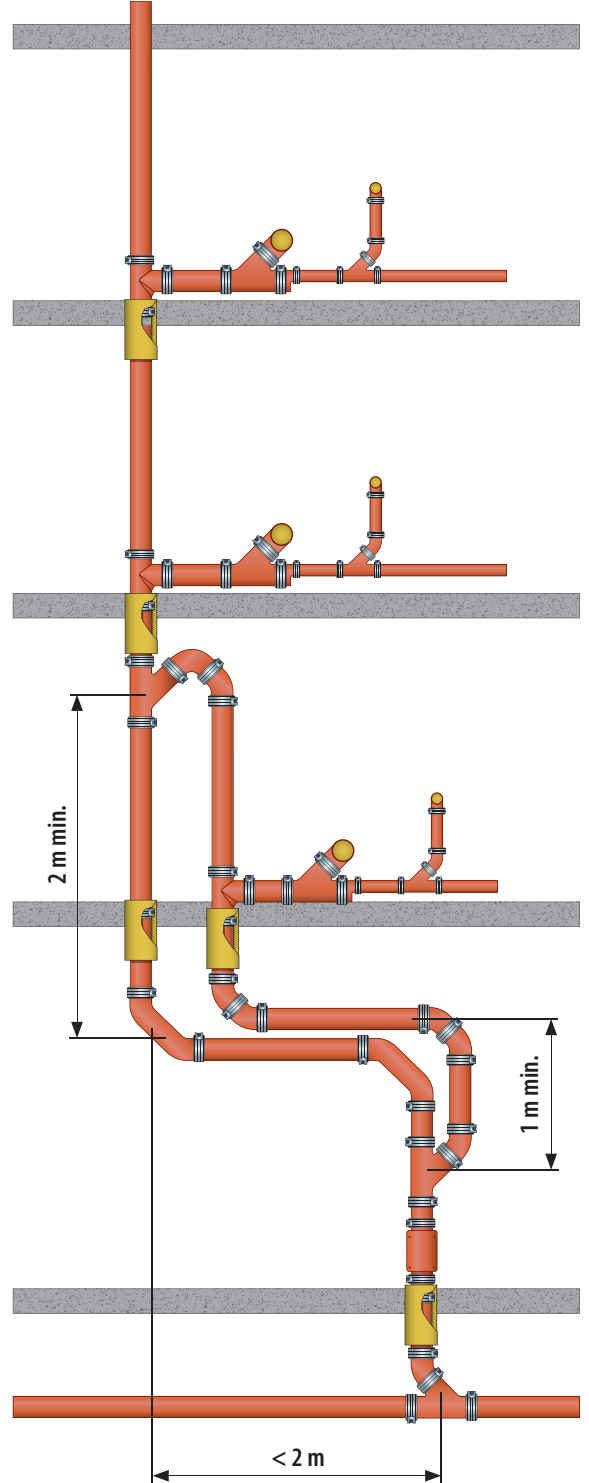
Resim 13 Dikey boru distorsiyonu < 2m bypass borulu
