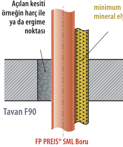
Resim 21 Yangından korunma açısından tavan boru hatları talepleri
